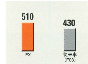
●フォーク上昇速度 (全負荷) ガソリン4.0トン比較 mm/sec
