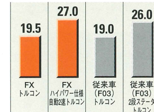
●走行速度 (無負荷) ディーゼル4.5トン比較 km/h
